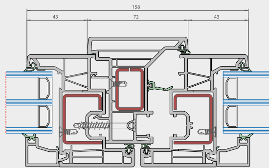
Horizontale snede
