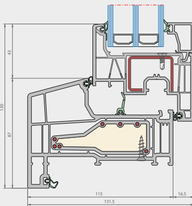
Verticale snede
